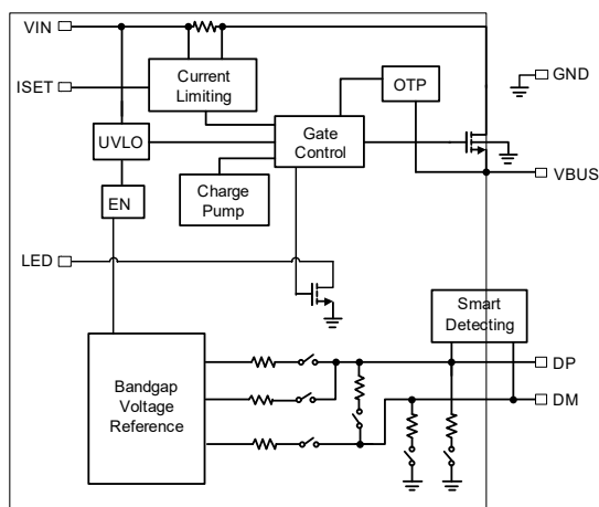
TX5601 功能框图
