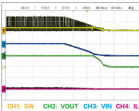
V_{IN}=24V V_{OUT}=5V 关闭波形 I_{OUT}=0A
