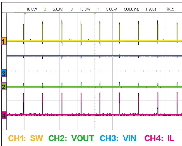
V_{IN}=12V V_{OUT}=5V 短路波形
