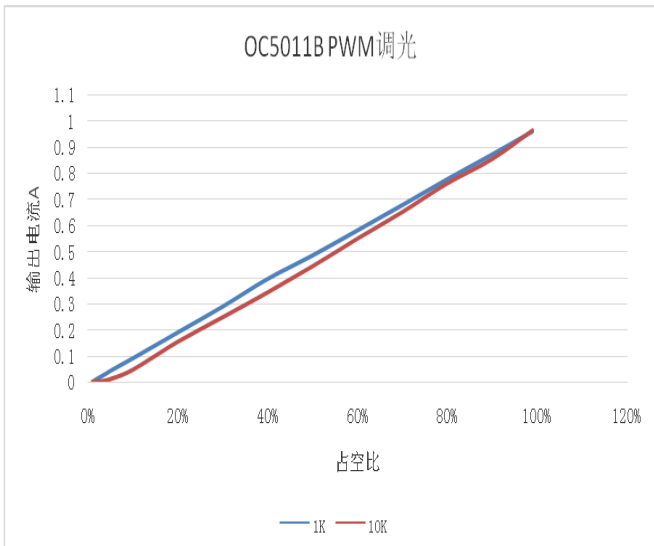
PWM 调光特性曲线
